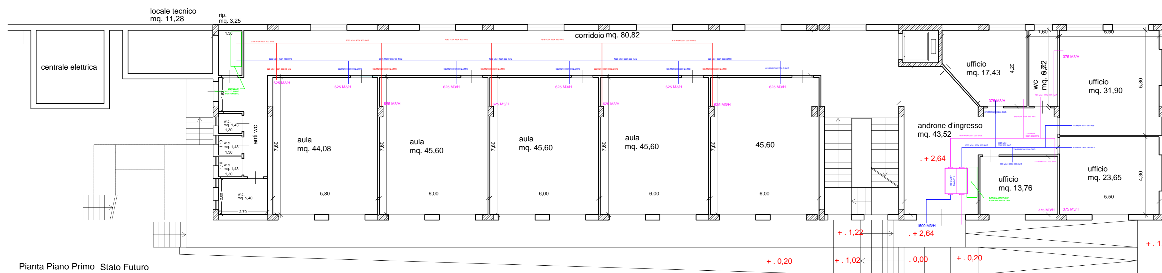
Impianto Trattamento Aria Planimetria Piano Primo
