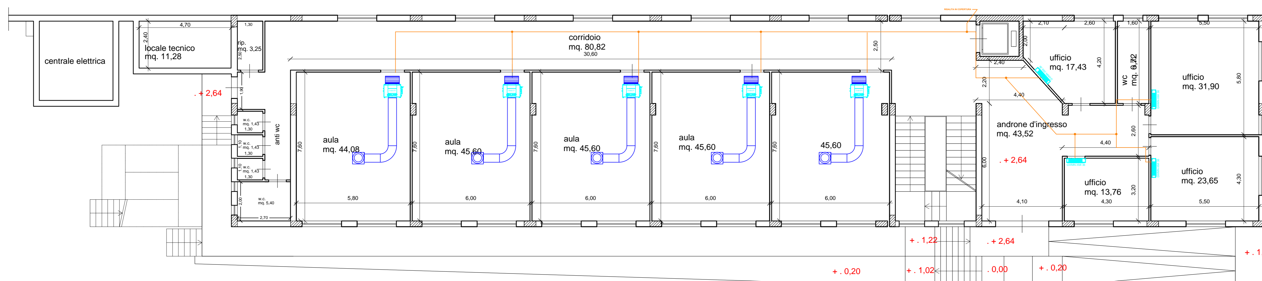
Impianto Clima Planimetria Piano Primo
