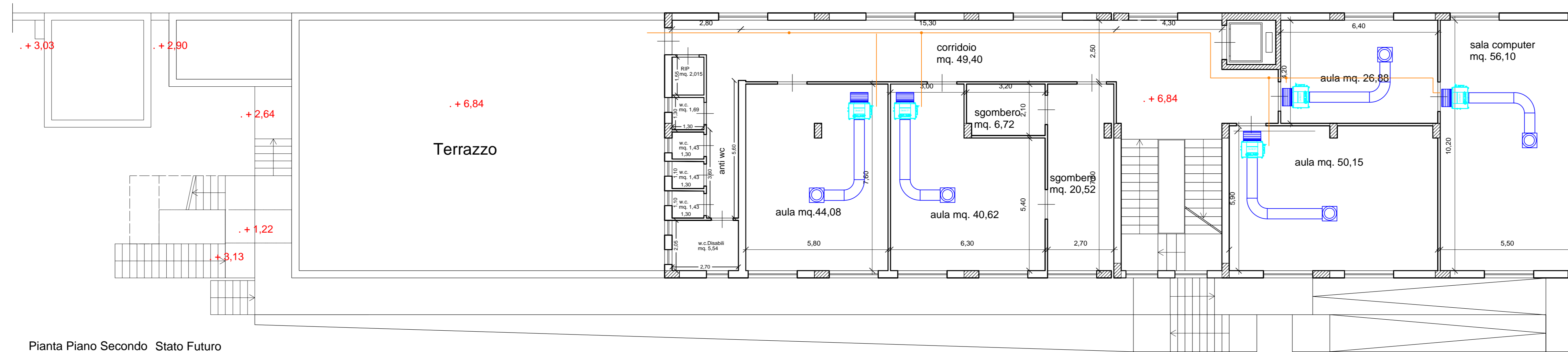
Pianta Piano Secondo Stato Futuro
